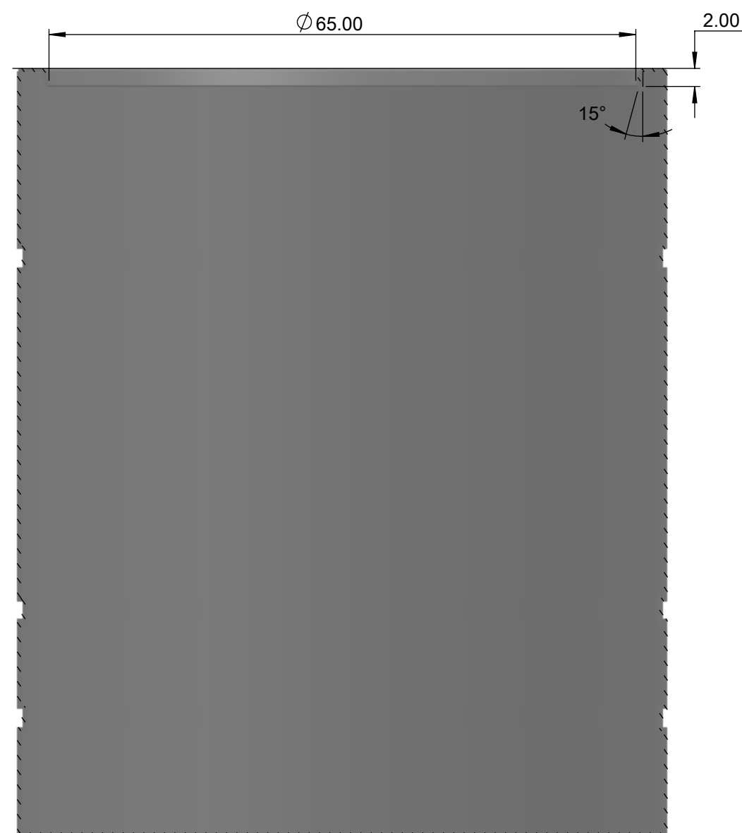
SECTION A-A
