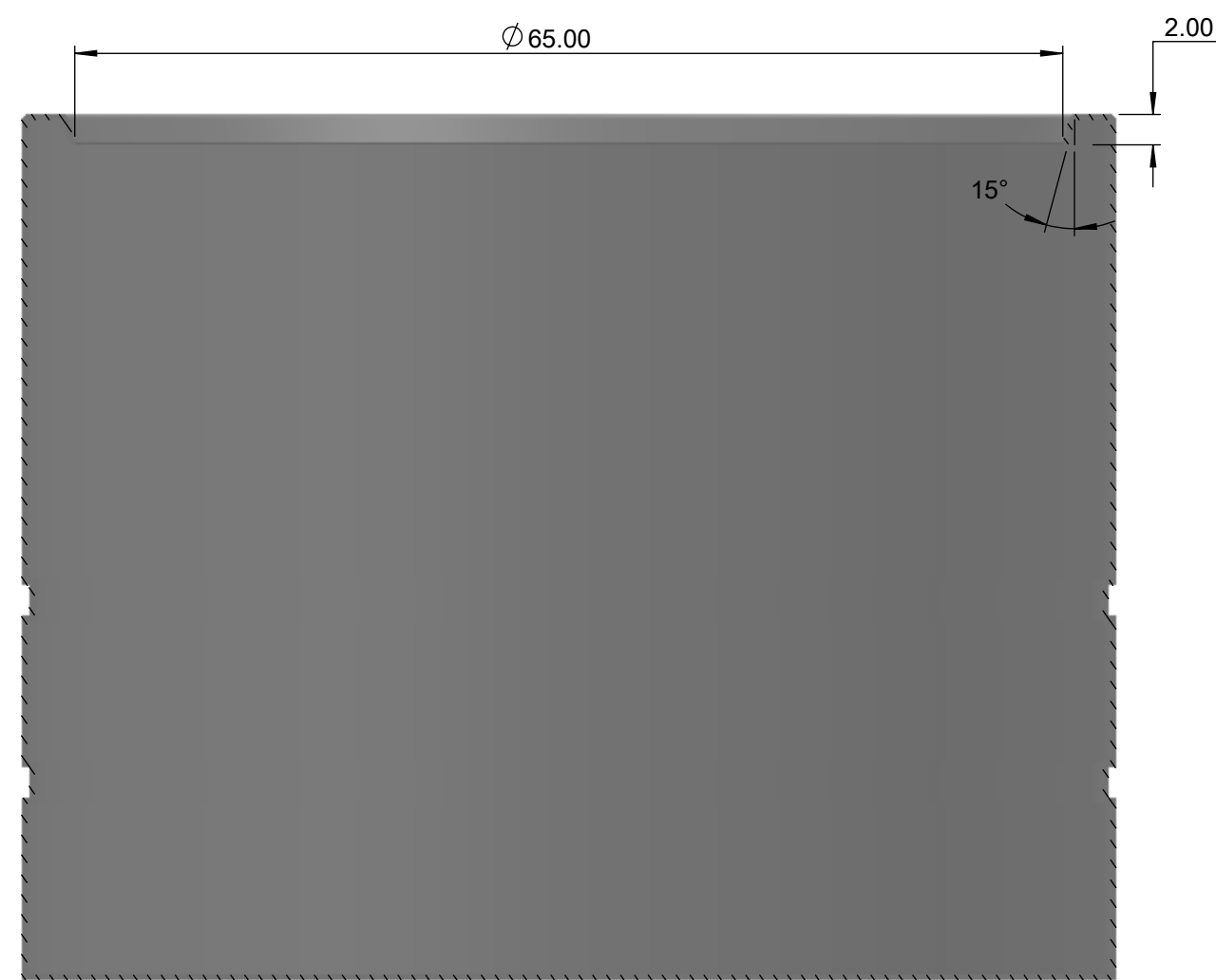
SECTION A-A
