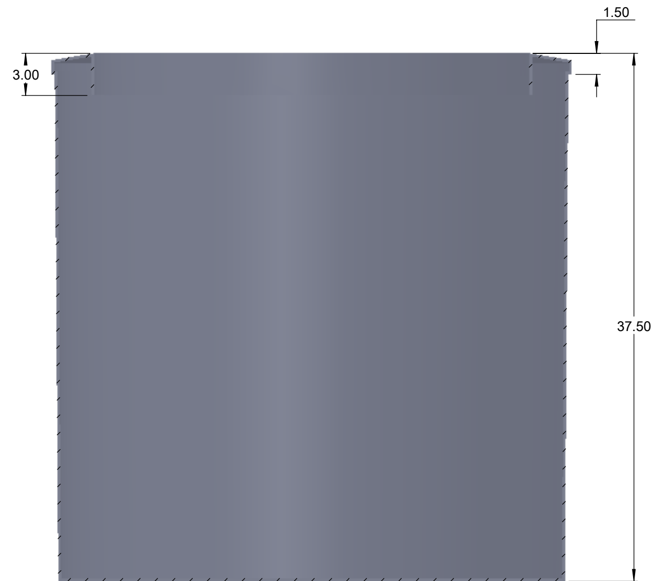
SECTION A-A
